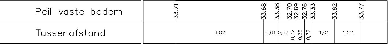
DWARSPROFIEL Vergelijkingsvlak 30.00 m T.A.W.
