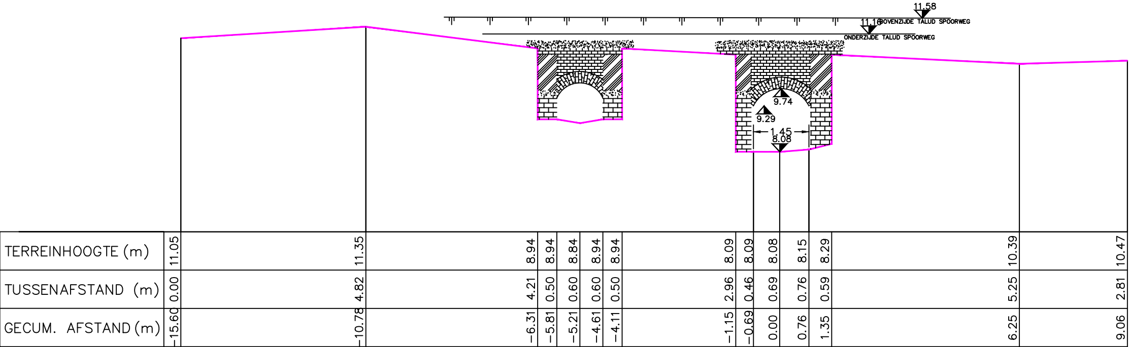
K170 VOORAANZICHT
