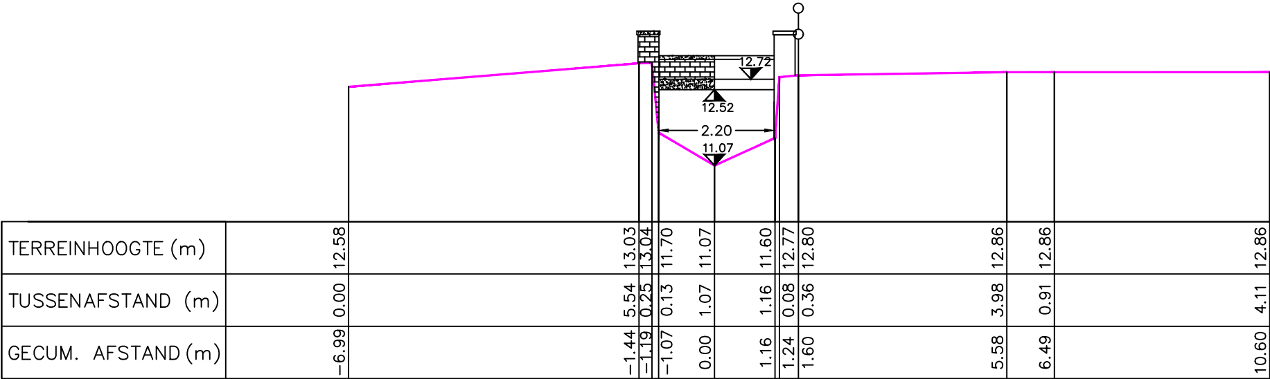
K270 VOORAANZICHT
