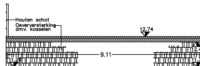
K310 LANGSDOORSNEDE
