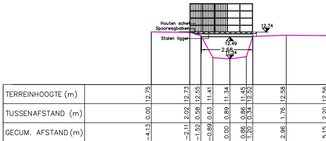
K310 VOORAANZICHT
