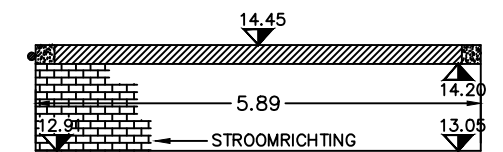
K340 LANGSDOORSNEDE
