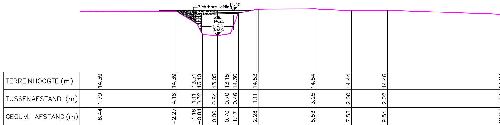
K340 VOORAANZICHT
