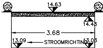
K350 LANGSDOORSNEDE
