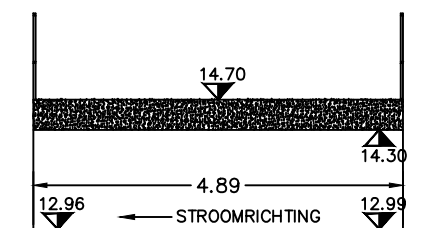
K360 VLANGSDOORSNEDE
