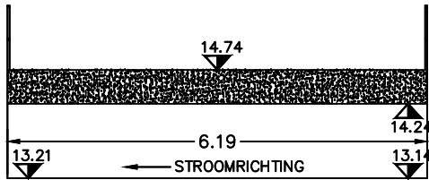
K380 LANGSDOORSNEDE
