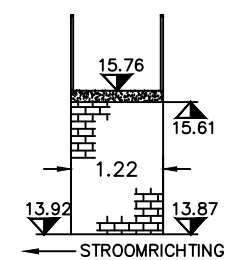
K390 LANGSDOORSNEDE
