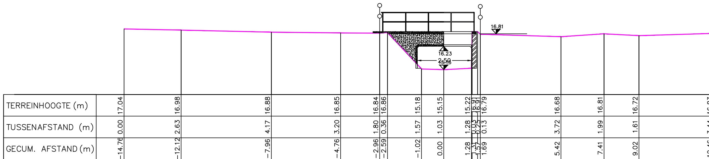
K430 VOORAANZICHT
