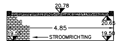
K490 VOORAANZICHT
