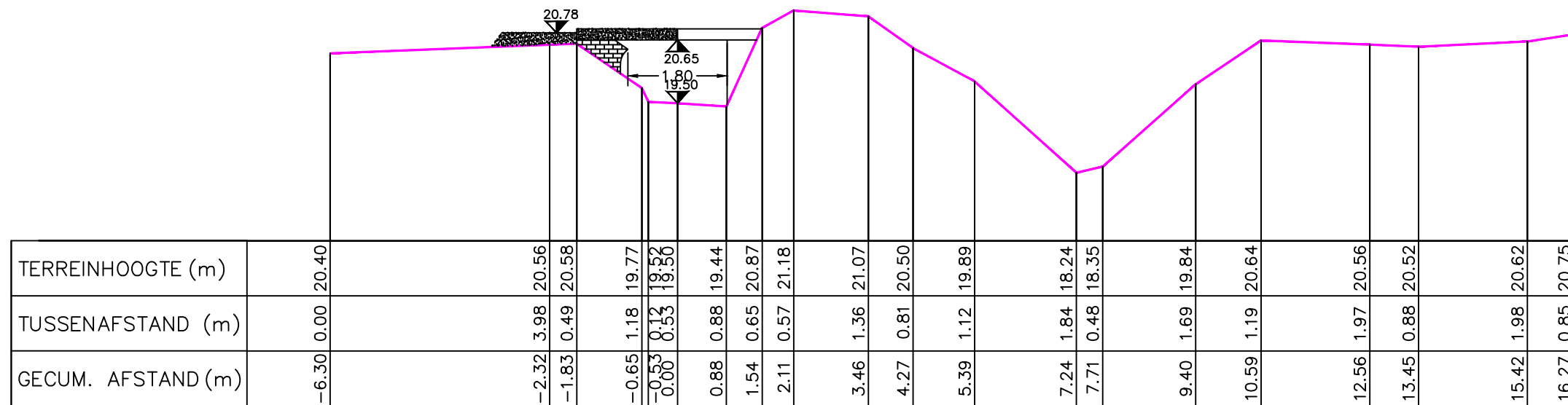
K490 VOORAANZICHT
