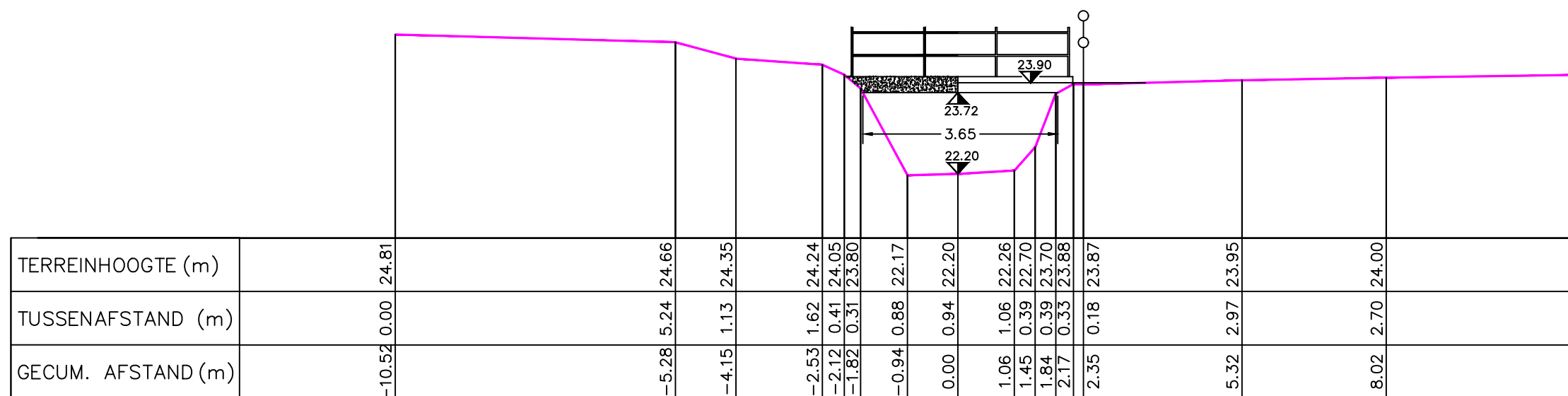
K510 VOORAANZICHT
