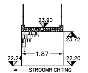
K510 VOORAANZICHT
