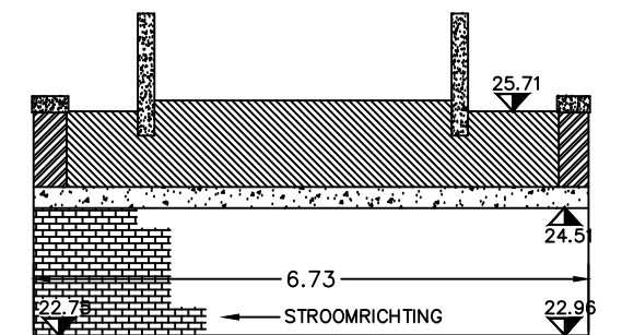
K530 LANGSDOORSNEDE
