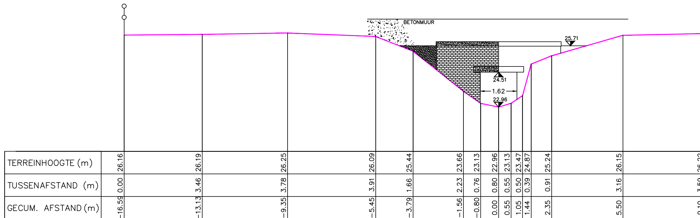
K530 VOORAANZICHT
