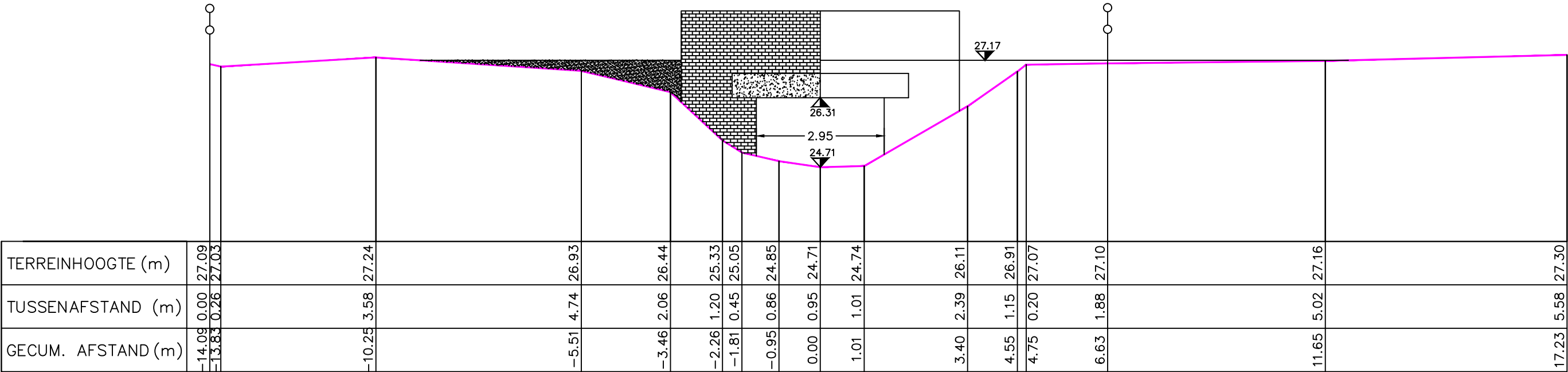
K540 VOORRAANZICHT
