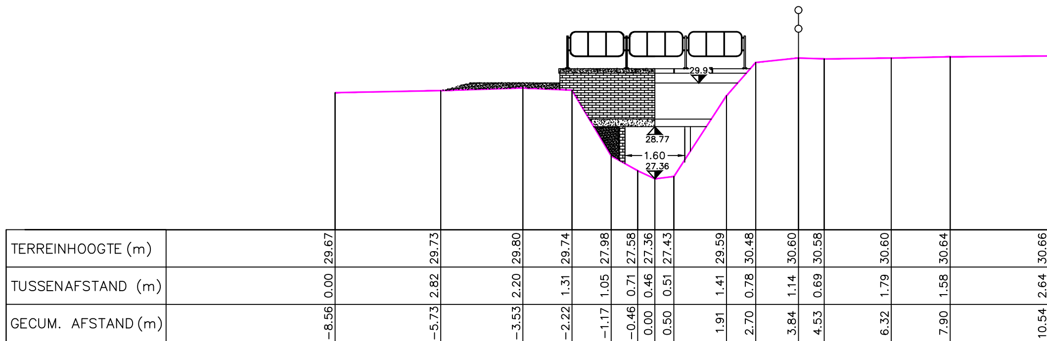
K570 VOORAANZICHT
