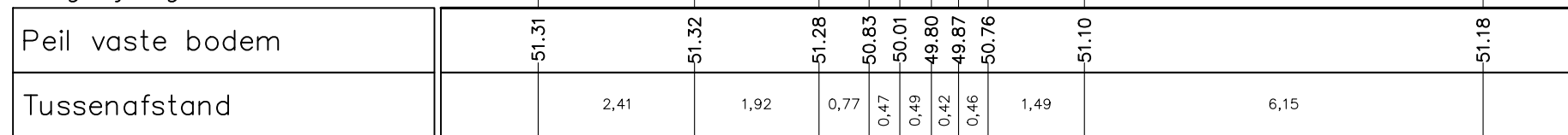
DWARSPROFIEL Vergelijkingsvlak 48.00 m T.A.W.
