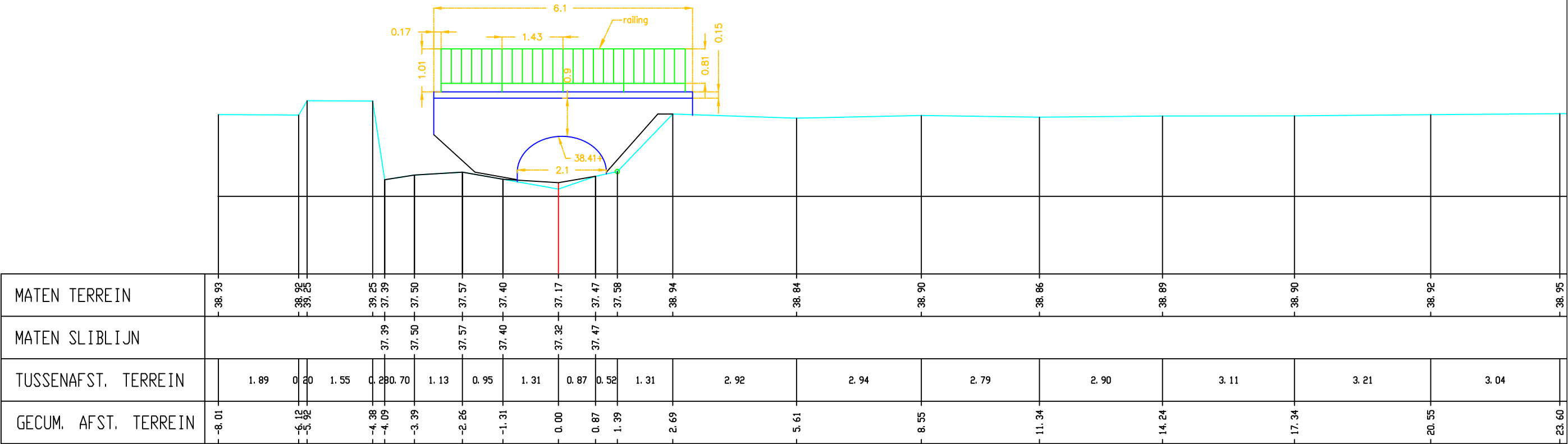
Kunstwerk 7156-441 (geprojecteerd haaks op as)
