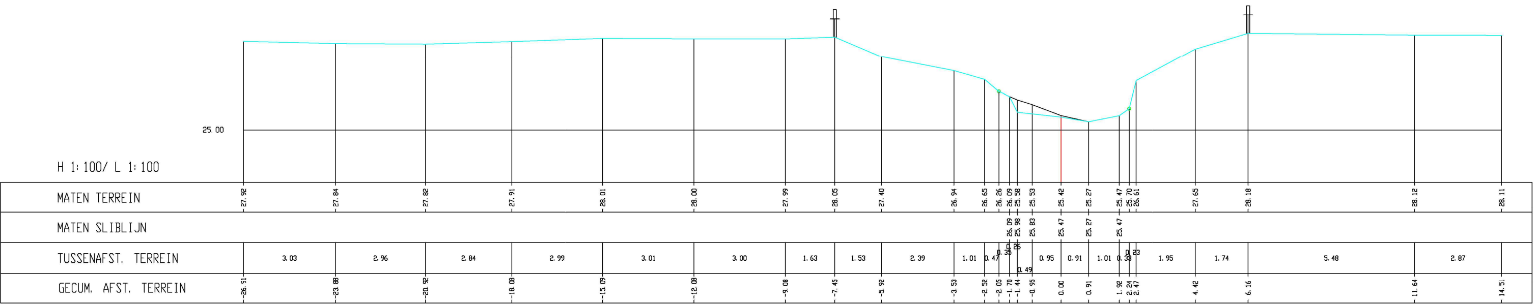
Vloedgracht, Dwarsprofiel 001
