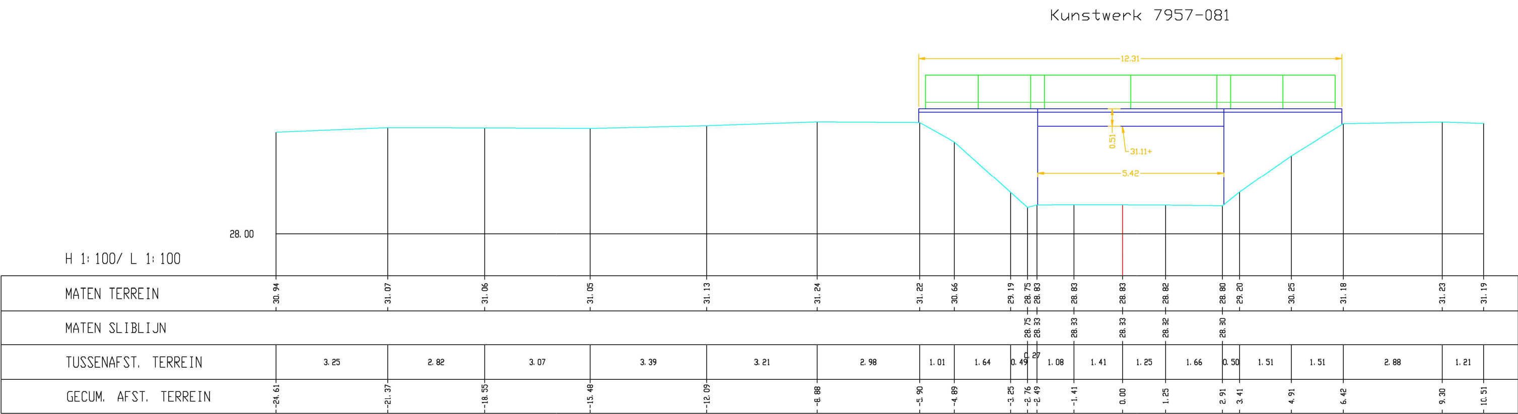
Vloedgracht, Dwarsprofiel 083
