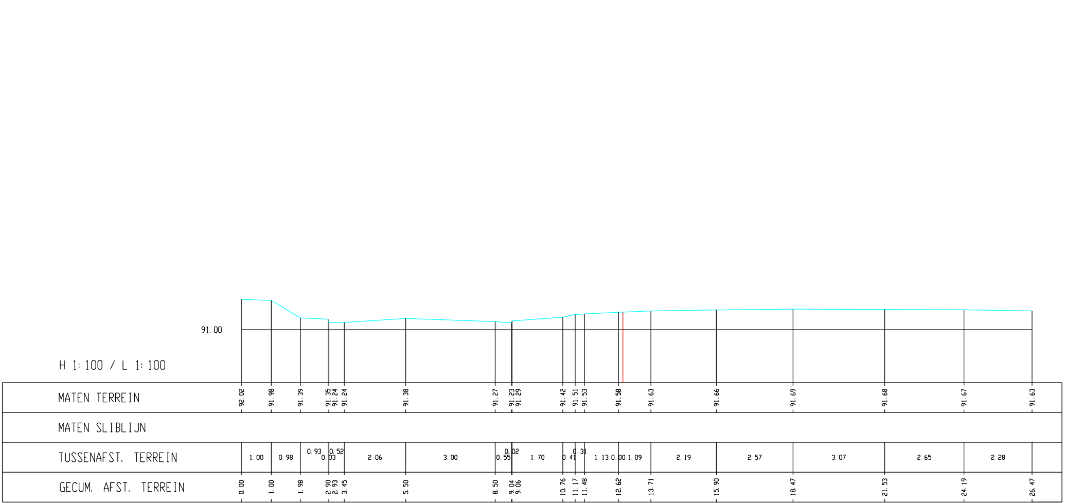
Voer, Molentak1,Dwarsprofiel K12
