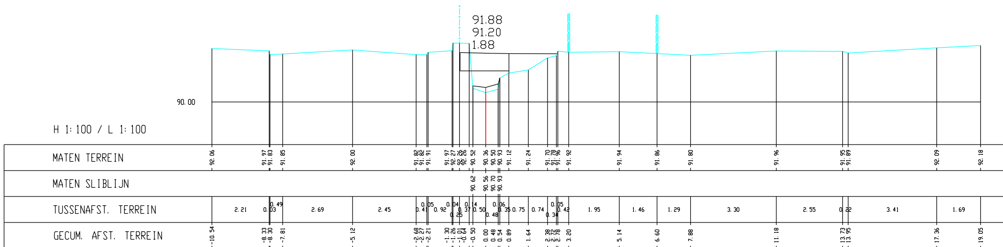
Voer, Molentak1, Dwarsprofiel K14
