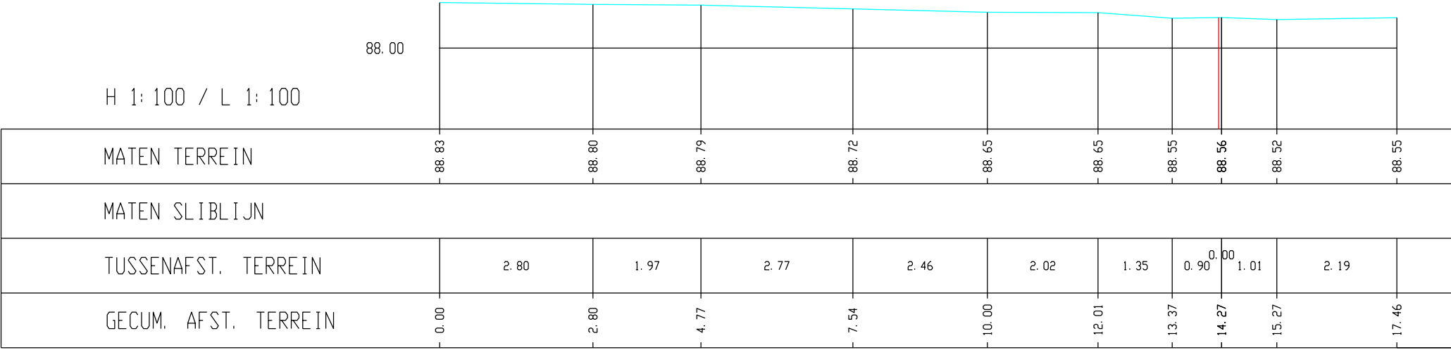
Voer, Molentak1,Dwarsprofiel K3
