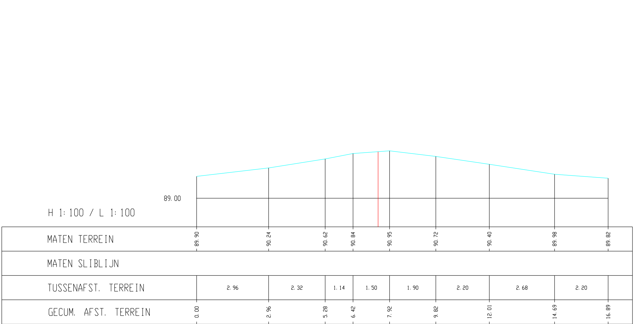
Voer, Molentak1,Dwarsprofiel K6
