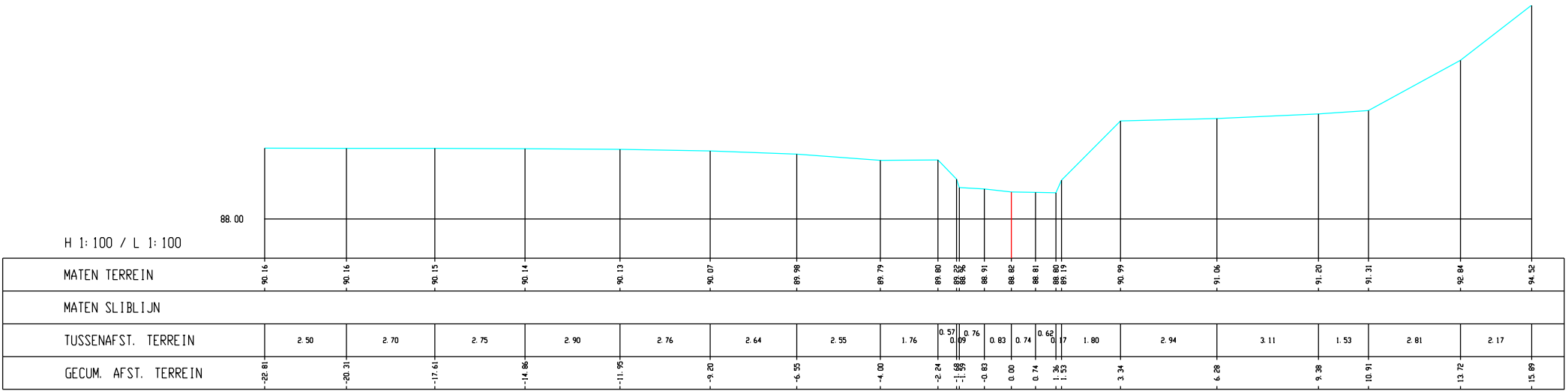
Voer, Dwarsprofiel K100
