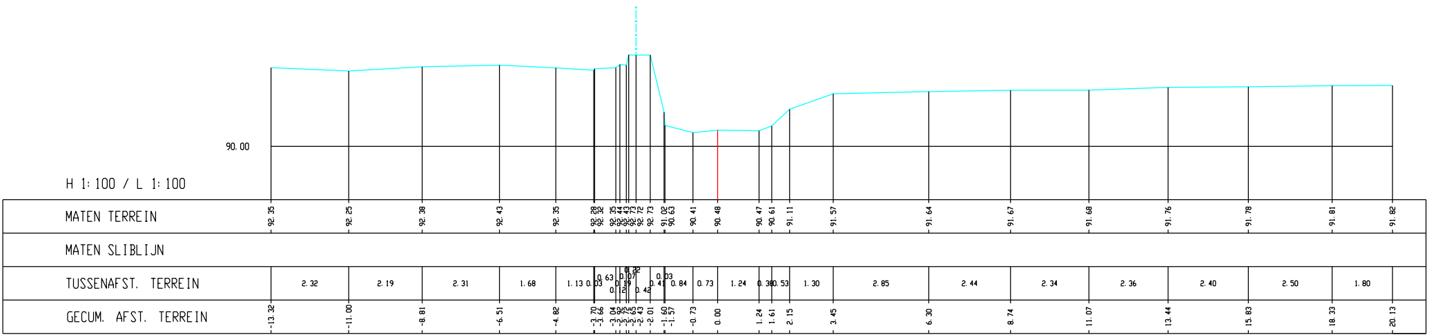
Voer, Dwarsprofiel K107
