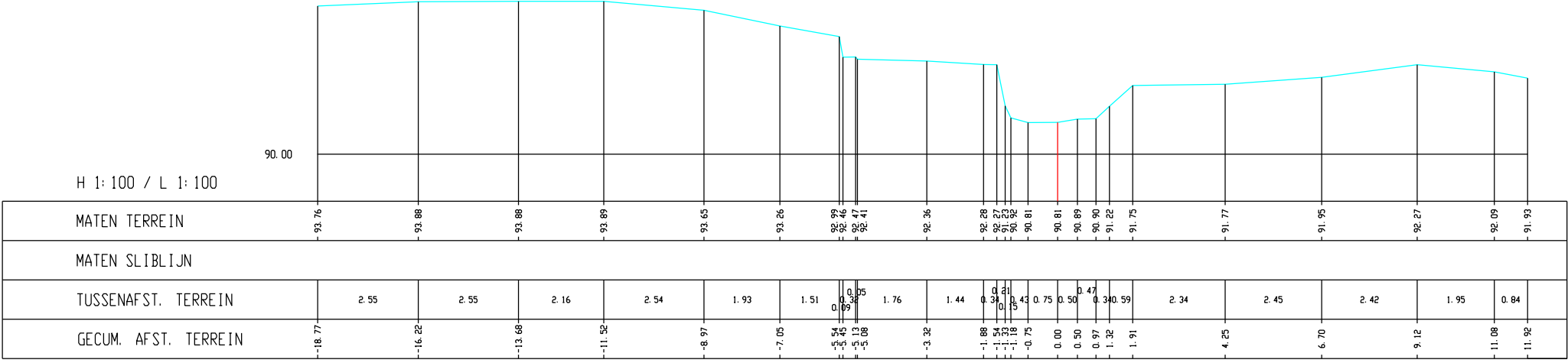
Voer, Dwarsprofiel K111
