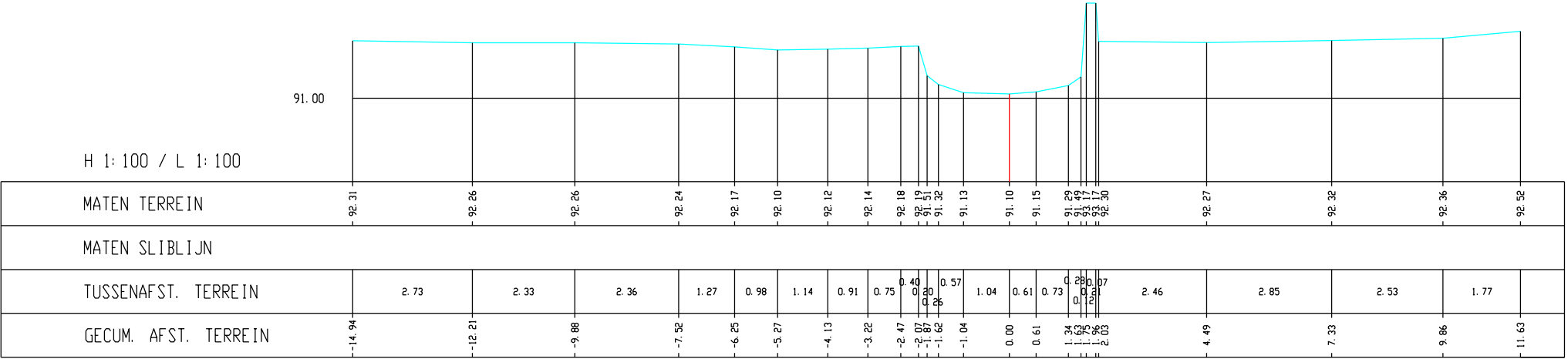
Voer, Dwarsprofiel K113
