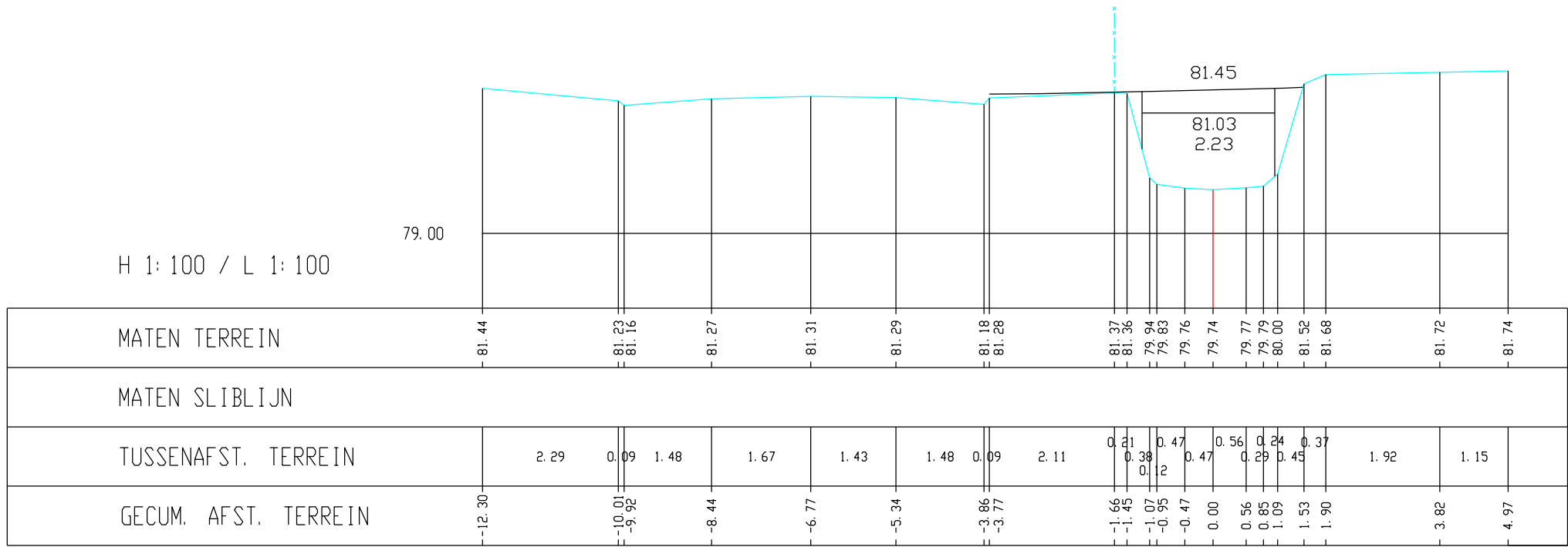
Voer, Dwarsprofiel K30
