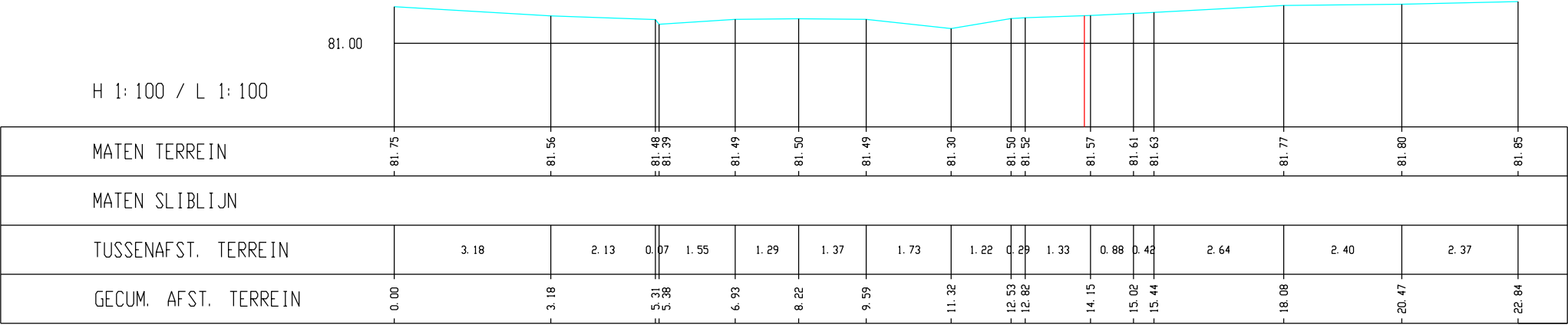
Voer, Dwarsprofiel K35
