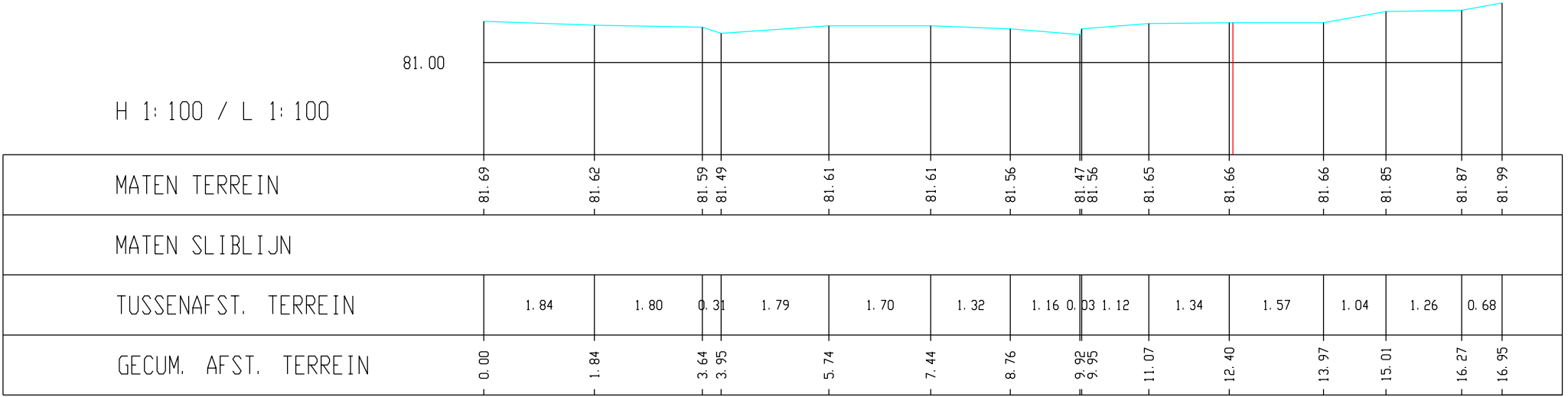
Voer, Dwarsprofiel K40
