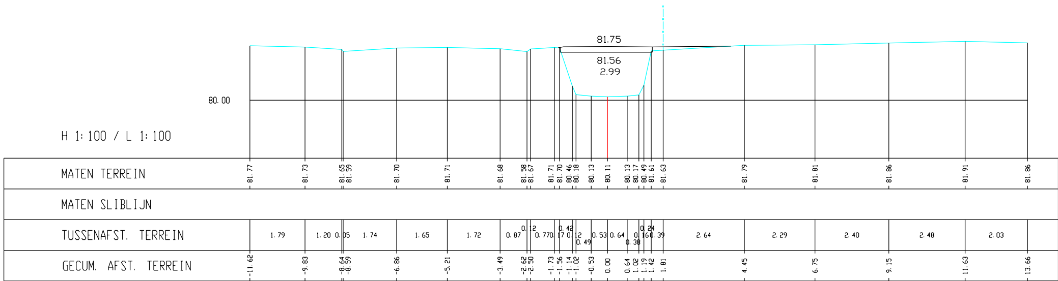
Voer, Dwarsprofiel K43
