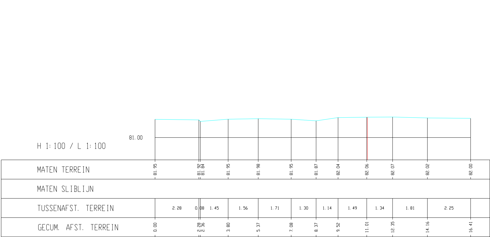
Voer, Dwarsprofiel K49
