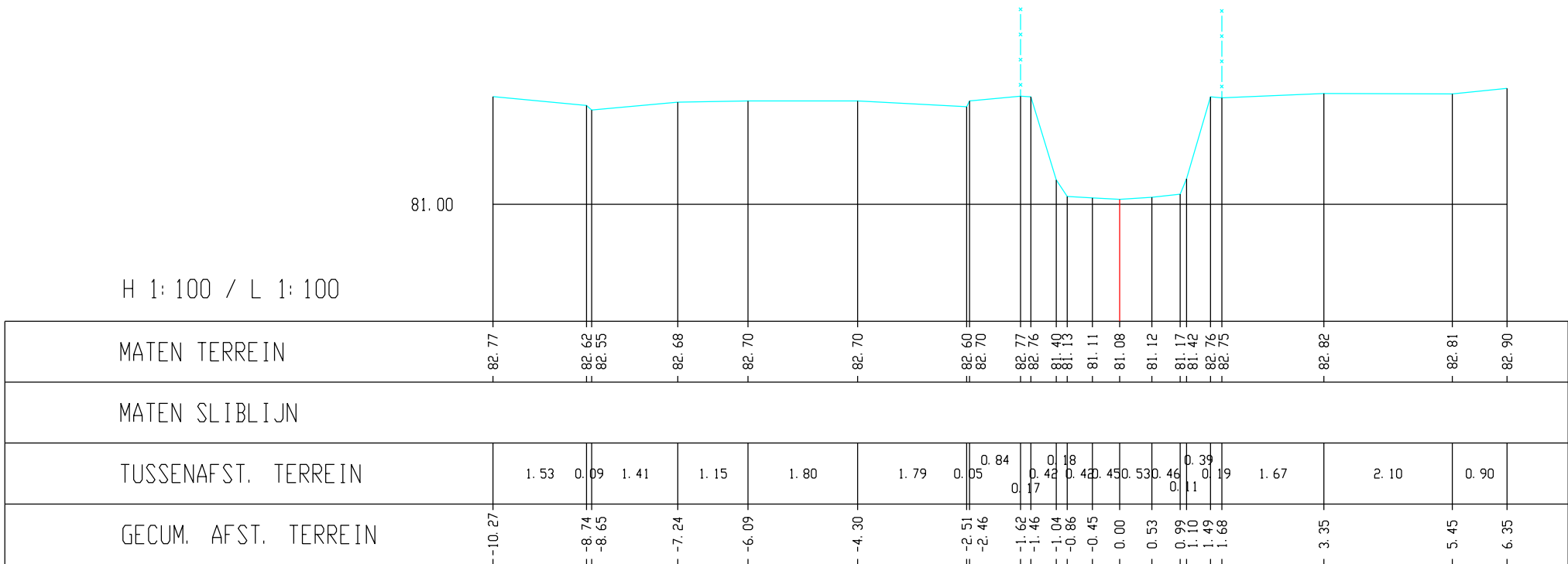
Voer, Dwarsprofiel K61
