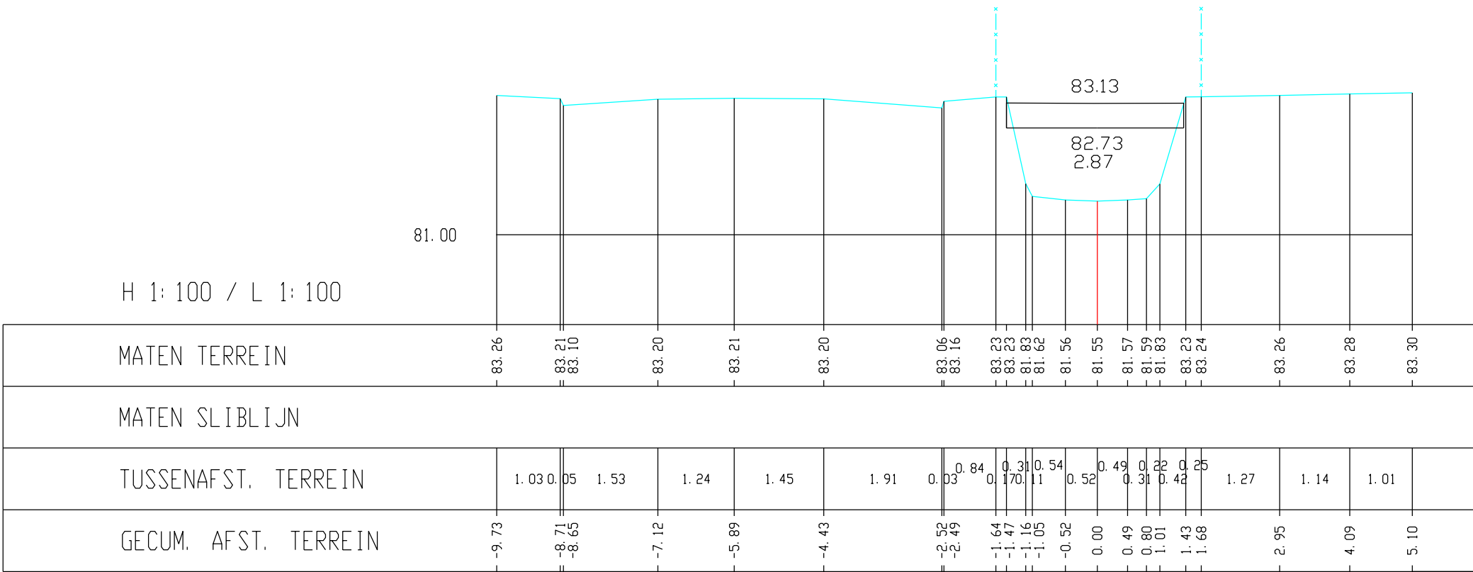
Voer, Dwarsprofiel K70
