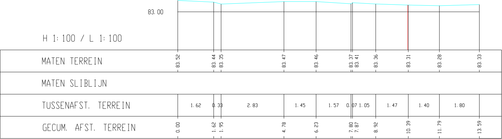
Voer, Dwarsprofiel K74
