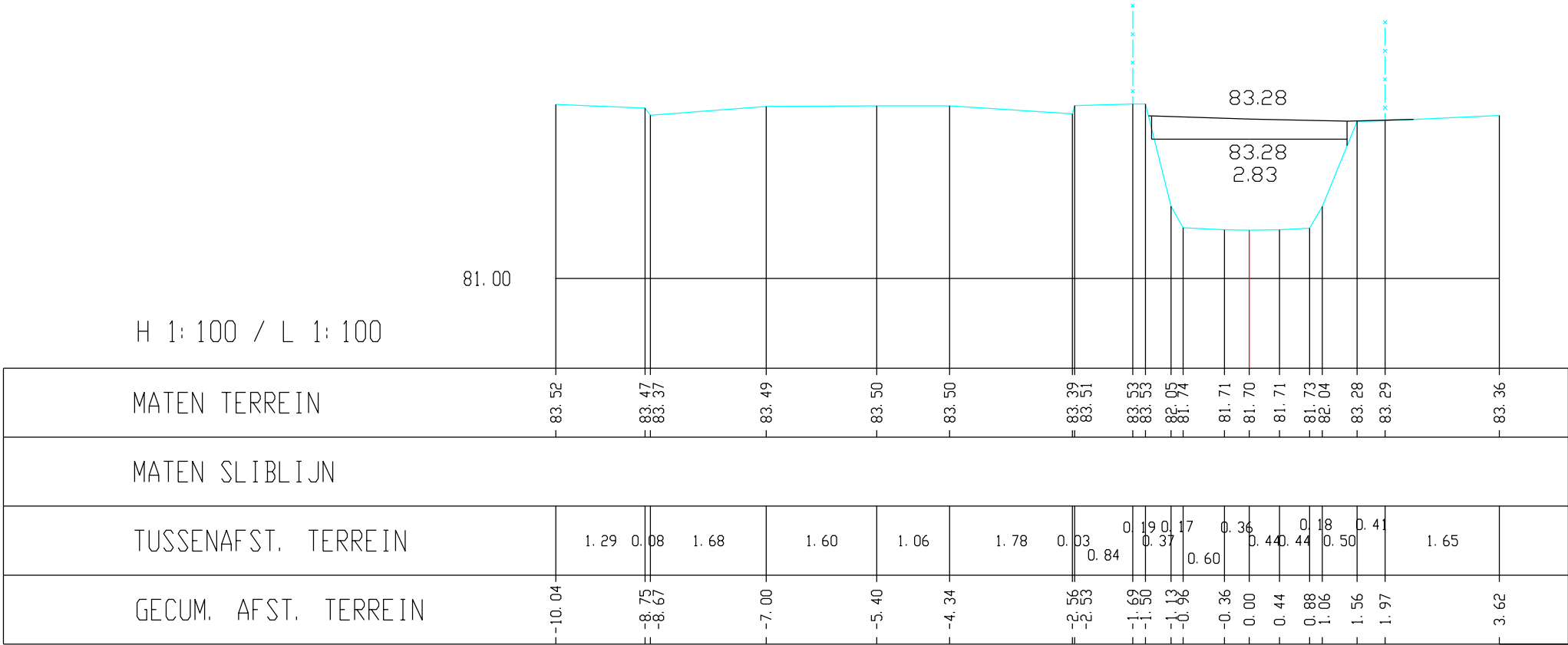
Voer, Dwarsprofiel K75
