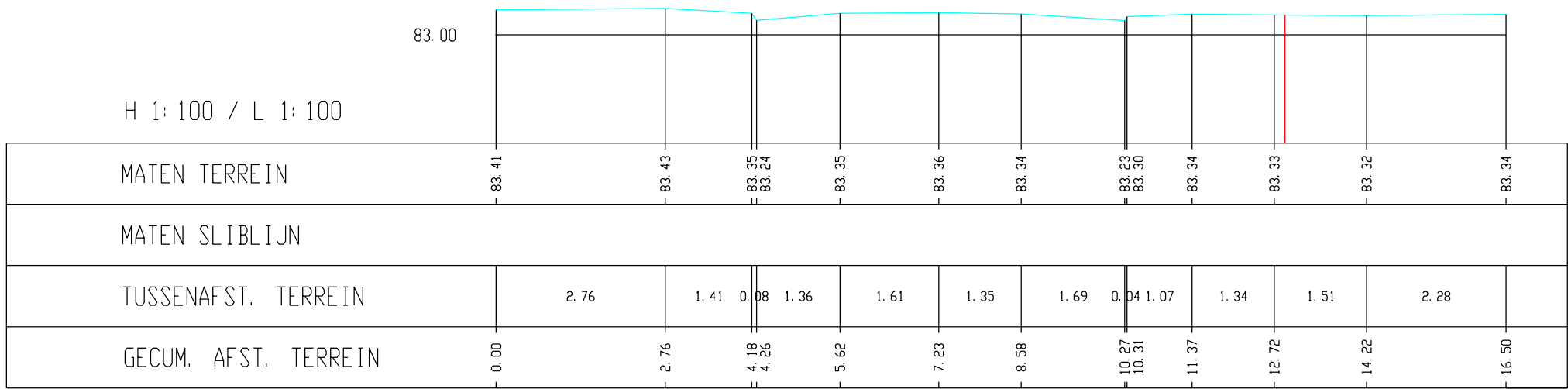
Voer, Dwarsprofiel K79
