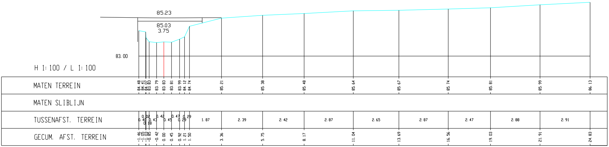
Voer, Dwarsprofiel K84
