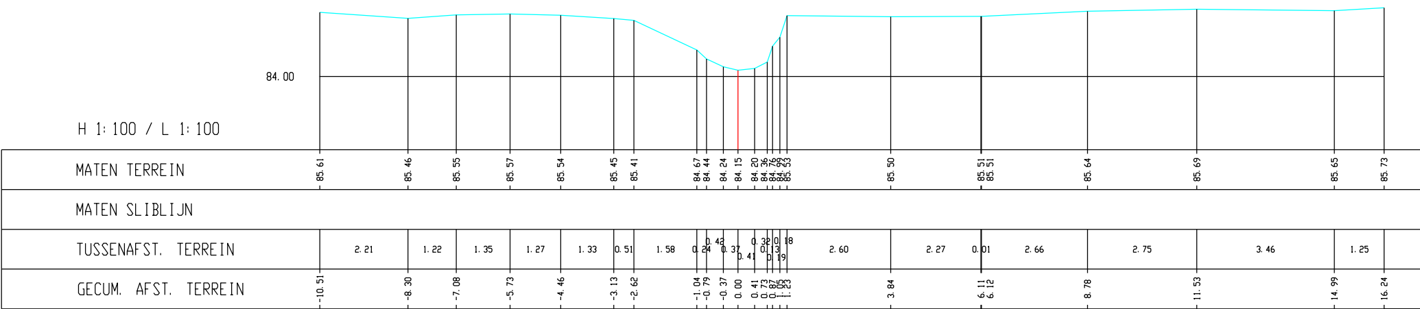
Voer, Dwarsprofiel K85
