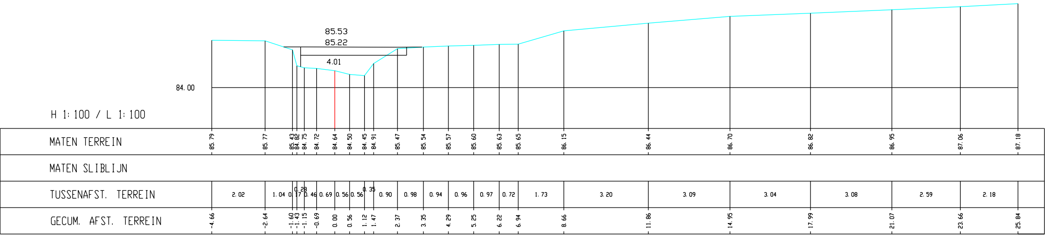
Voer, Dwarsprofiel K87
