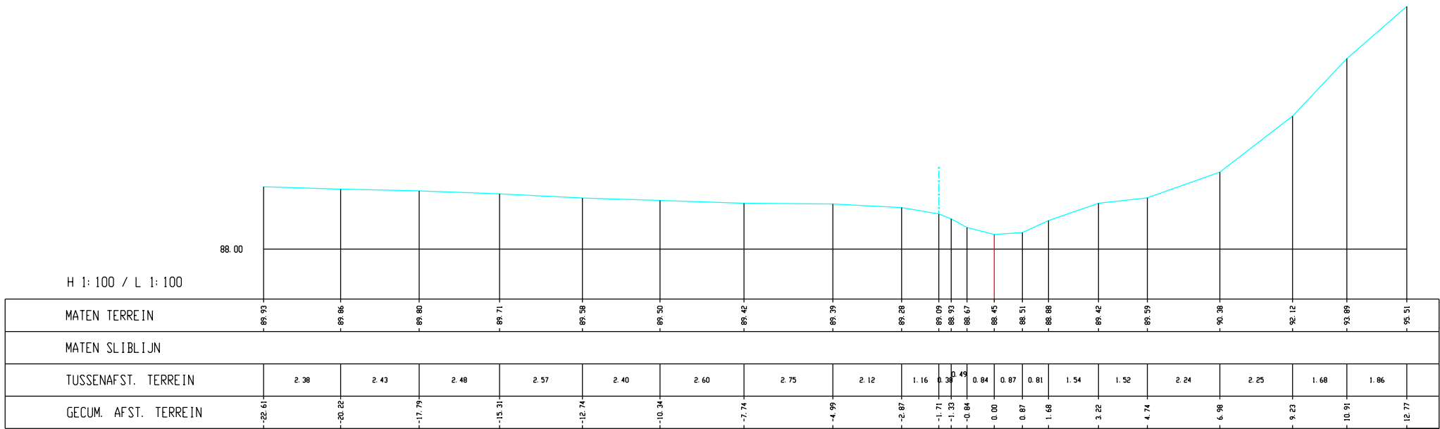
Voer, Dwarsprofiel K99
