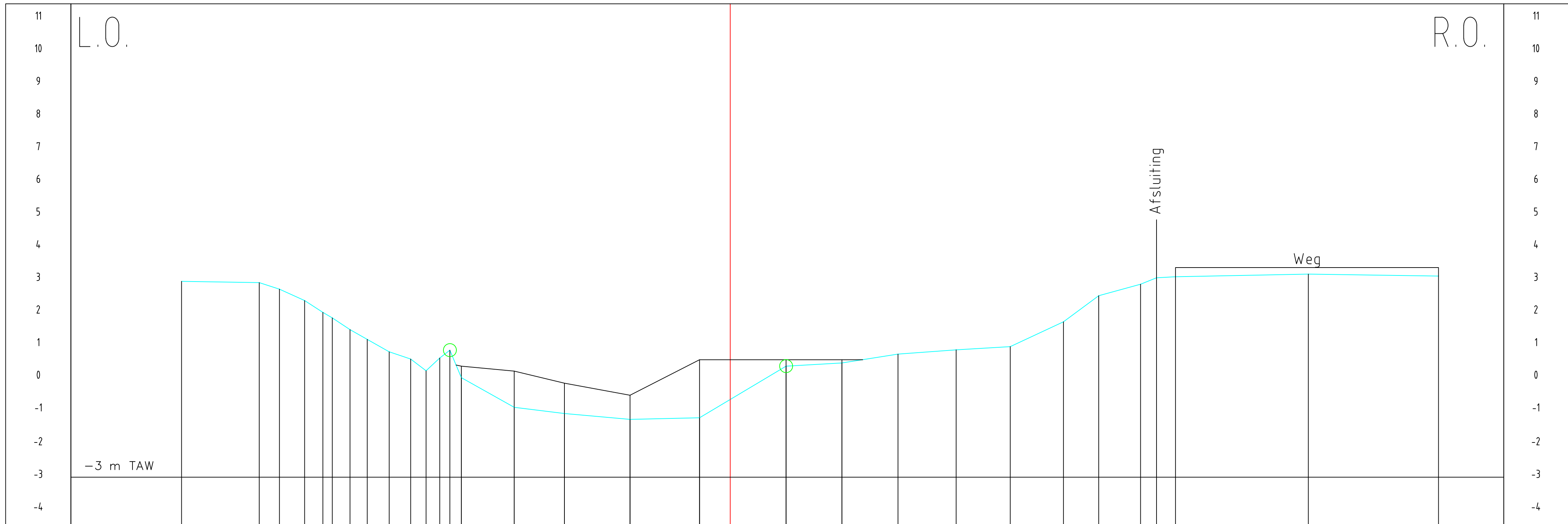
Profiel 35
