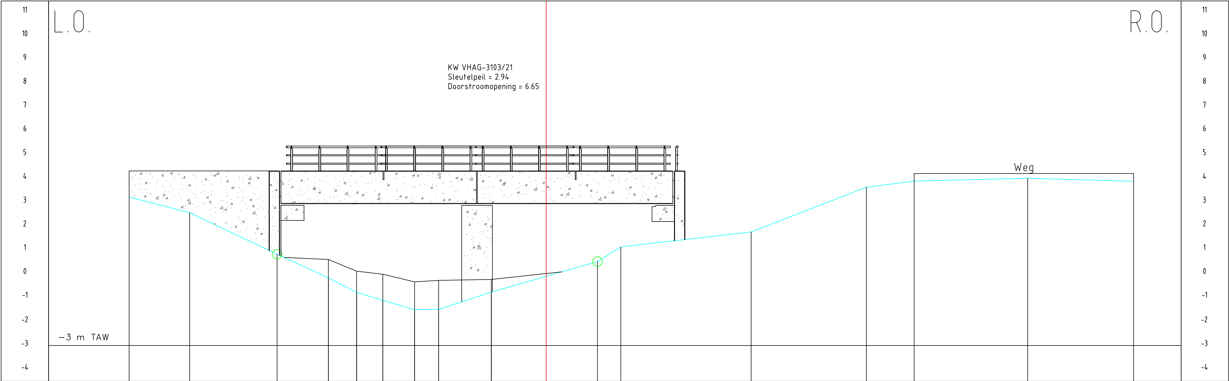
Profil 46
