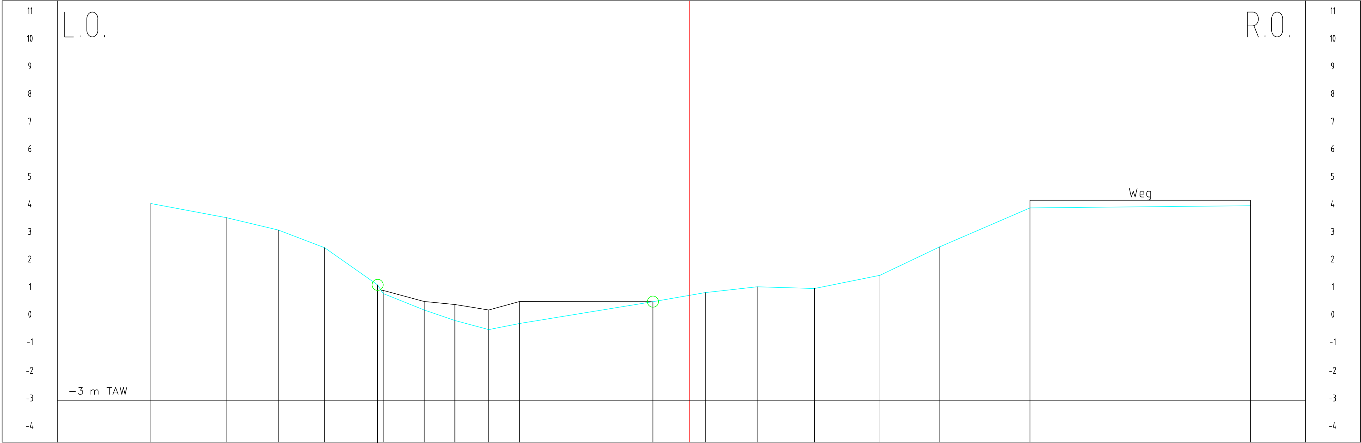
Profiel 89
