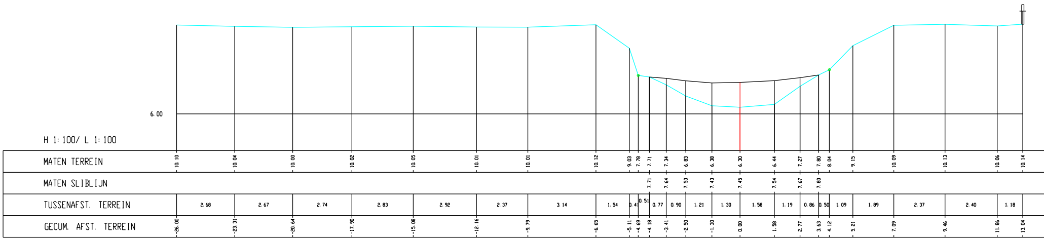
Wimp, Dwarsprofiel 123
