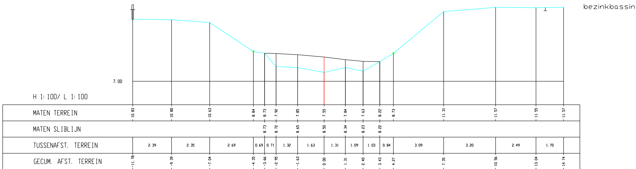
Wimp, Dwarsprofiel 143
