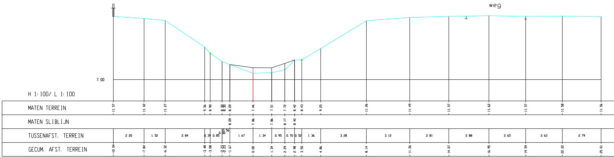
Wimp, Dwarsprofiel 145
