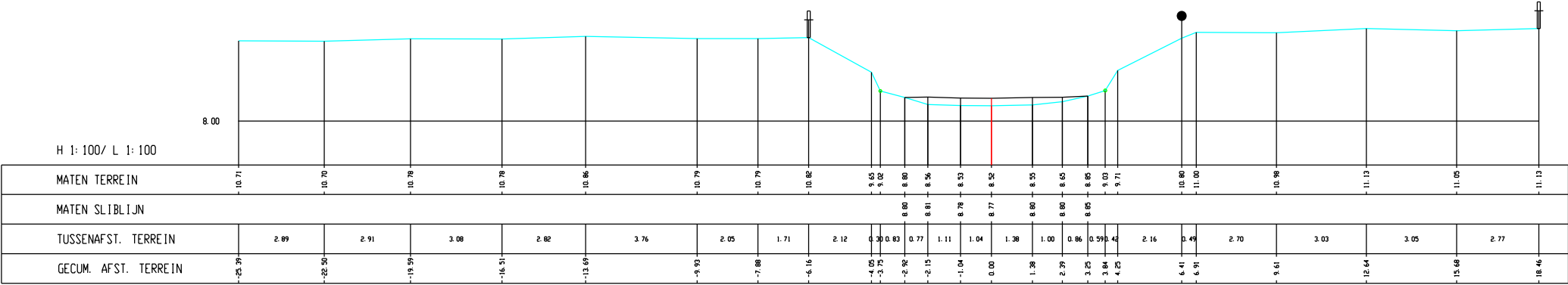
Wimp, Dwarsprofiel 158
