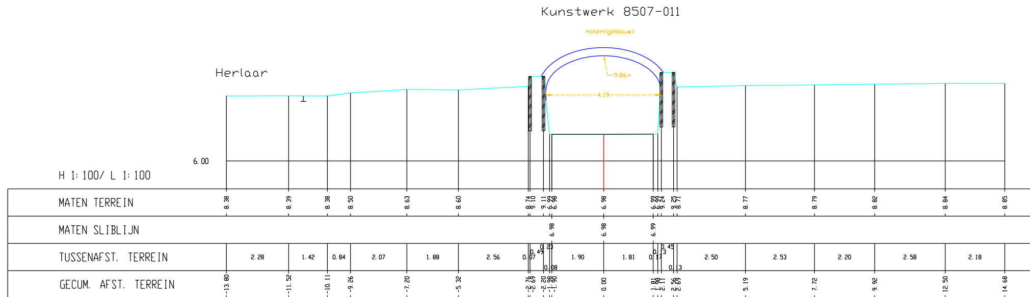
Wimp, Dwarsprofiel 023
