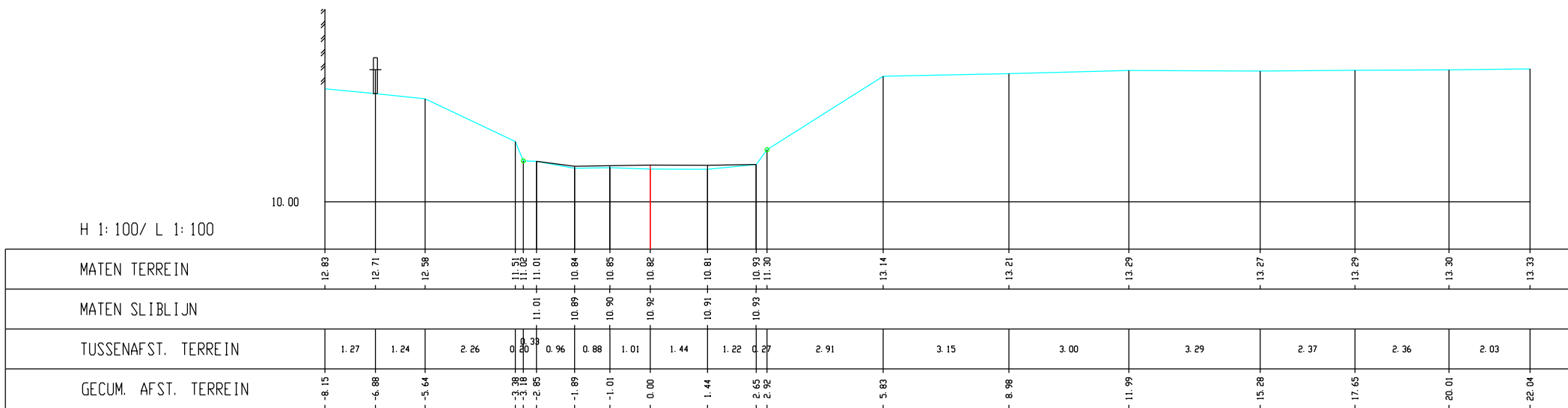
Wimp, Dwarsprofiel 231
